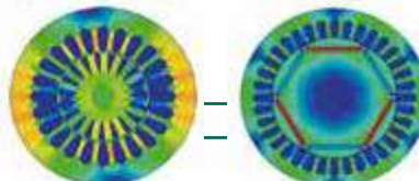
Motor Inducción Motor Imanes
